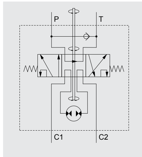
Dirección Hidrostática DHS-3000 SENSIBLE
