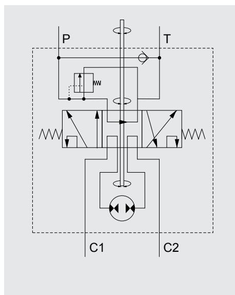
Dirección Hidrostática DHS-V 3000 SENSIBLE C/LIMITADORA DE PRESION
