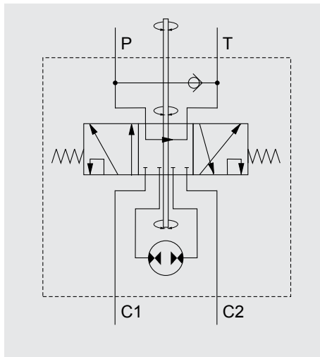
Dirección Hidrostática DHI-3000 INSENSIBLE
